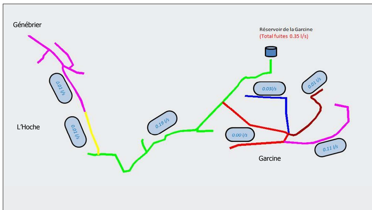
Figure 32 : Répartition des écoulements nocturnes par tronçon- réseau de la Garcine
