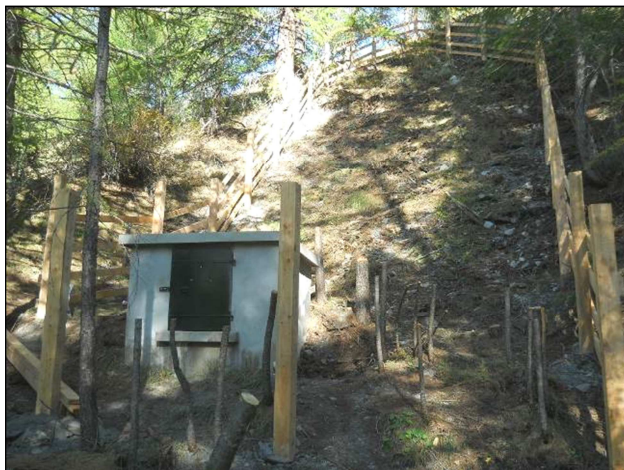
Photo 5 : Aspect extérieur du captage - Mounal 3 (Source : HYDRETTUES le 6 oct. 2011)
