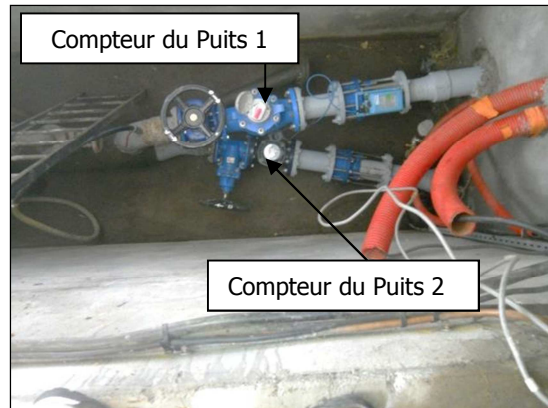
Photo 24 : Compteur des pompages (Source : HYDRETTUES le 15 Jul. 2013)
