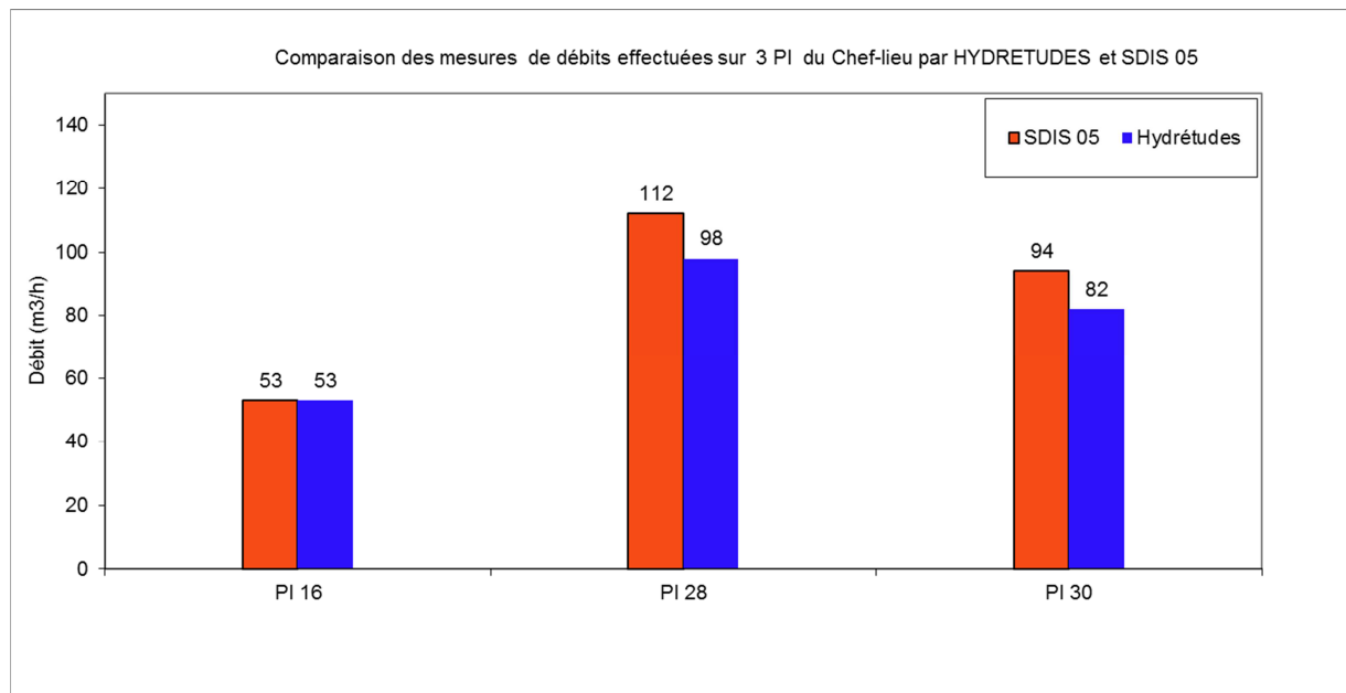
Figure 24 : Comparaison des mesures de débits effectuées sur 3 PI du Chef-lieu par HYDRETUDES et SDIS 05
